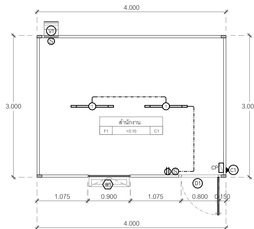
แบบแปลนพื้น
