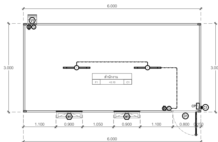
1 แบบแปลนพื้น SO-631 3.00x6.00x2.40 M.
