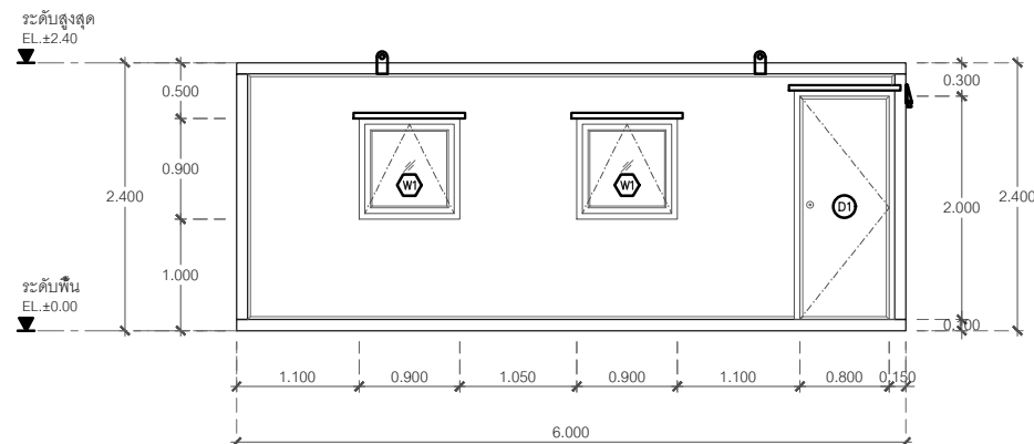
1 แบบรูปด้าน 1 ขนาดจริง 1:75
